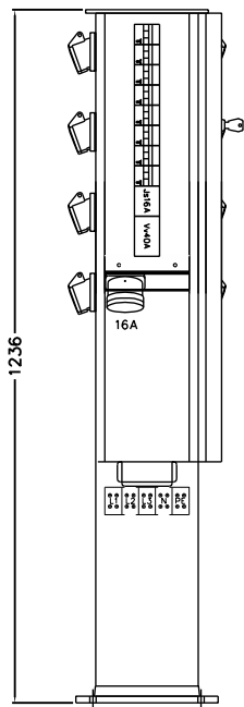
KÄYTTÖOVI AVATTUNA
