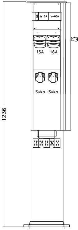
KÄYTTÖOVI AVATTUNA
