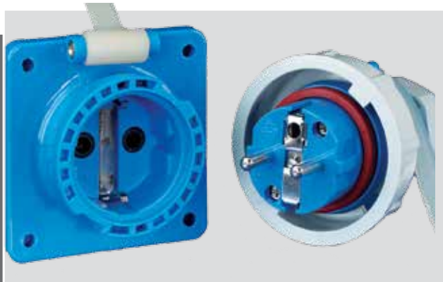
socket-outlet IP68
